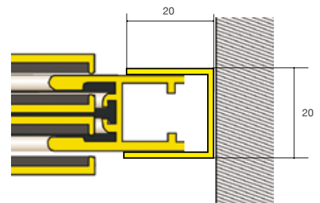
SEZ. ORIZZONTALE CON COMPENSATORE
