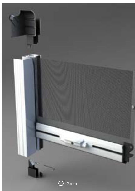
AGGANCIO INF. MANIGLIA CRICCHETTO
